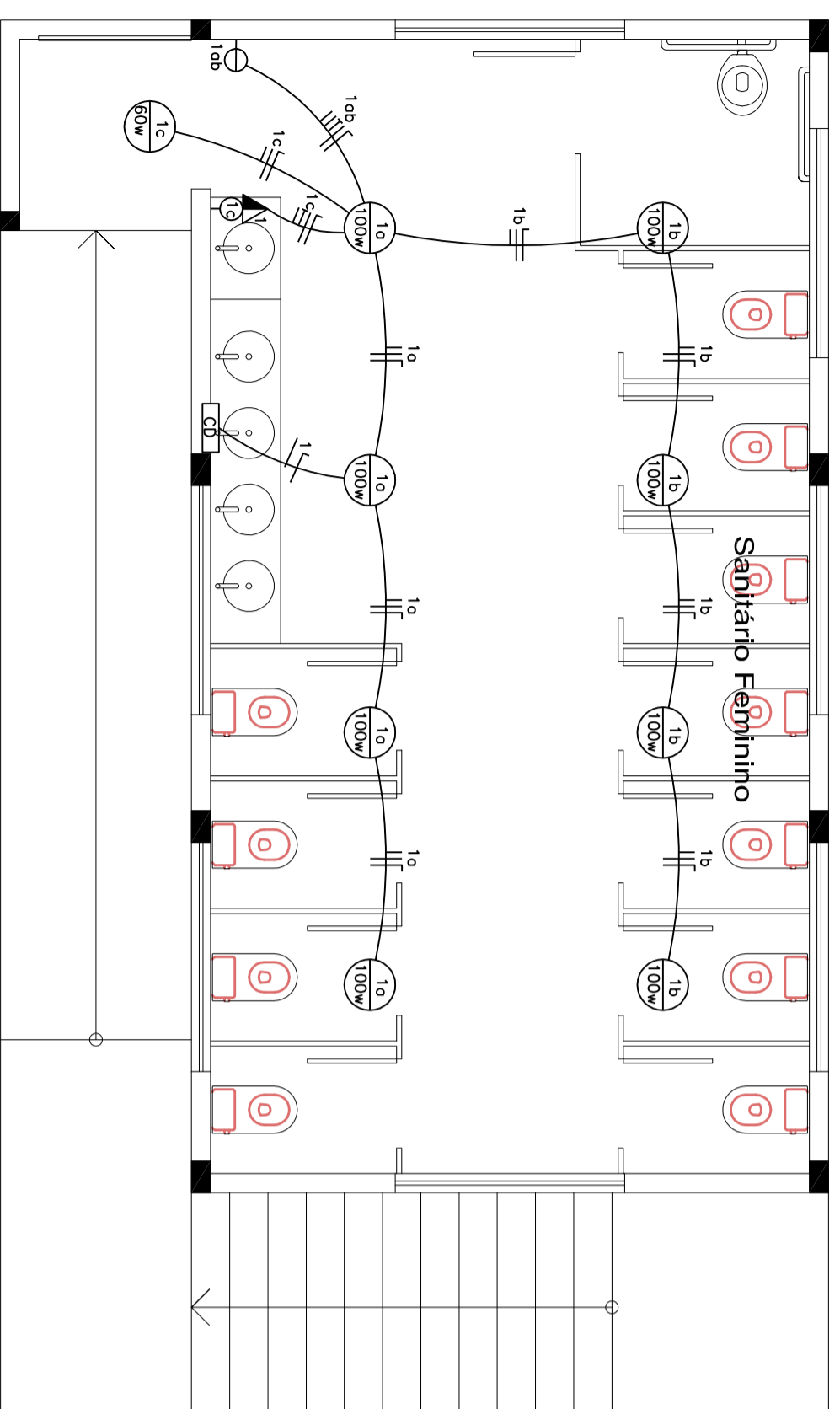
Inst. Elétrica - Sanit. Feminino
