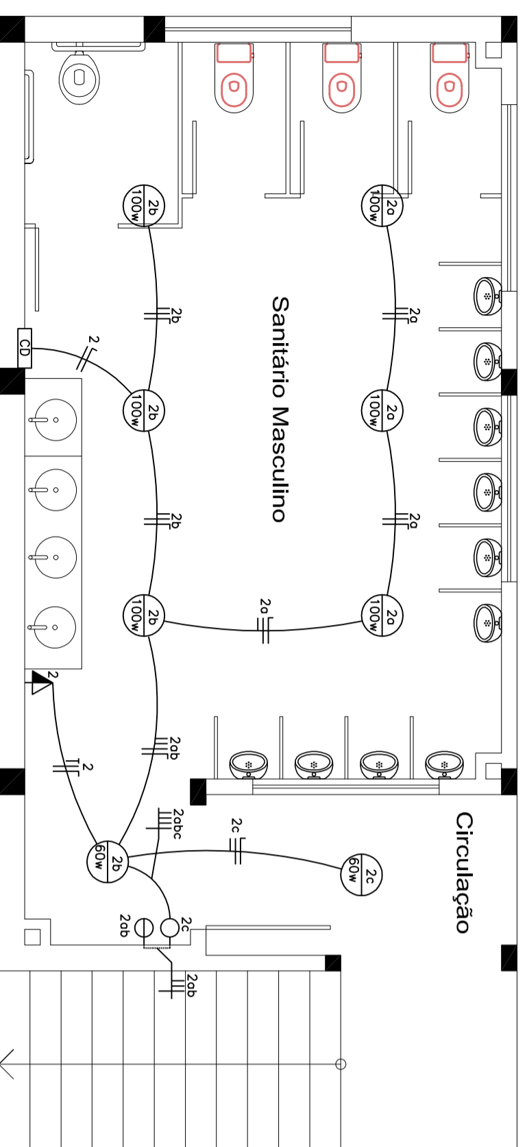
Planta Baixa - Sanit. Masculino
